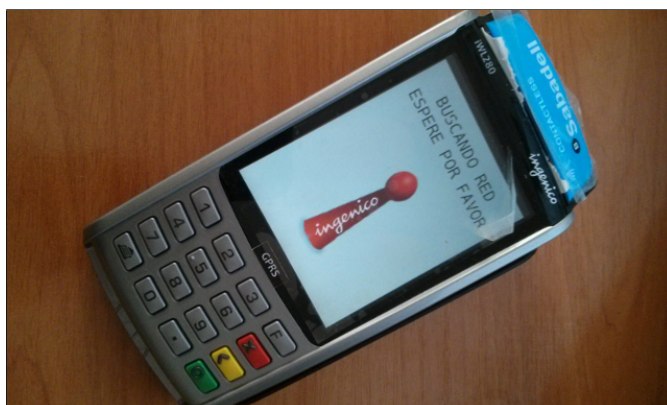
Figura 4.8: TPV Ingenico IWL280; GPRS y NFC.
