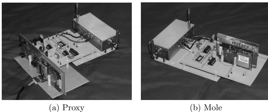
Figura 5.1: Hardware ad-hoc para implementar ataque de relay NFC.
